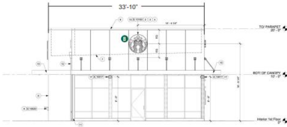
2 WEST ELEVATION Scale: 1/8" = 1'-0"
