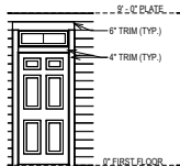
ENTRY DETAIL "C" SCALE: 1/8" = 1'-0"
