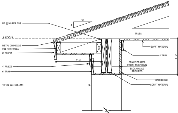
DTL - CORNICE DETAIL "C" SCALE: 1" = 1'-0"
