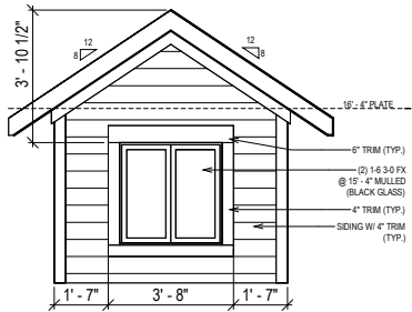
DORMER DETAIL "C" SCALE: 1/4" = 1'-0"
