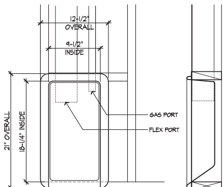
FRONT SIDE DRYER BOX DETAIL SCALE: N.T.S.
