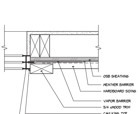
WINDOW JAMB
