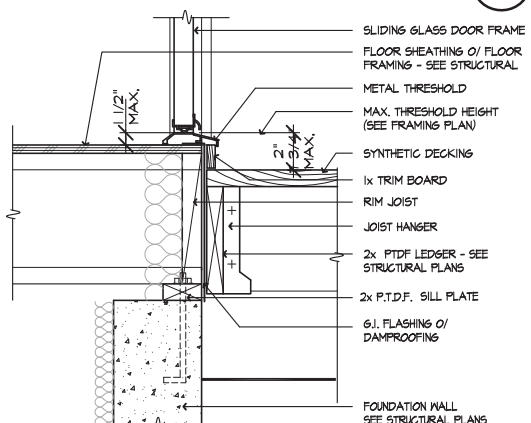
SWING DOOR THRESHOLD SCALE 1 1/2"=1'-0" 0820-01c
