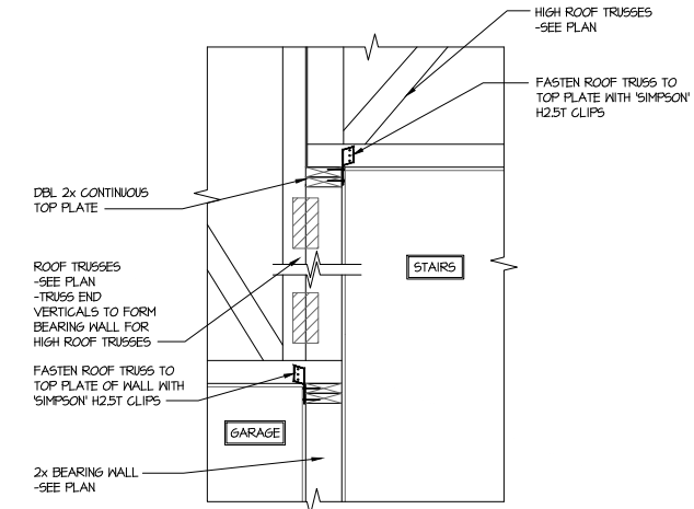
5 DETAIL SCALE: 3/4"=1'-0"
