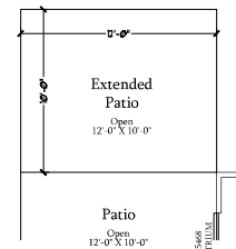
Optional Extended Patio
