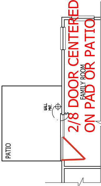
OPT. PATIO
