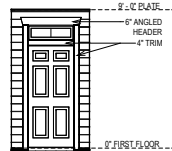
ENTRY DETAIL "B" SCALE: 1/8" = 1'-0"
