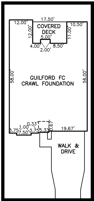
INSET SCALE: 1"=30"
