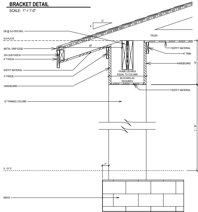
CORNICE DTL. SCALE: 1" = 1'-0"
