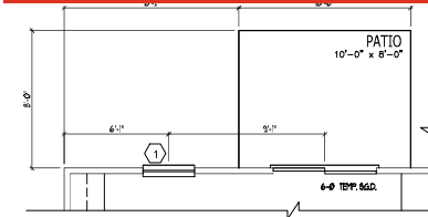
OPT PATIO SCALE: 1/4" = 1'-0"
