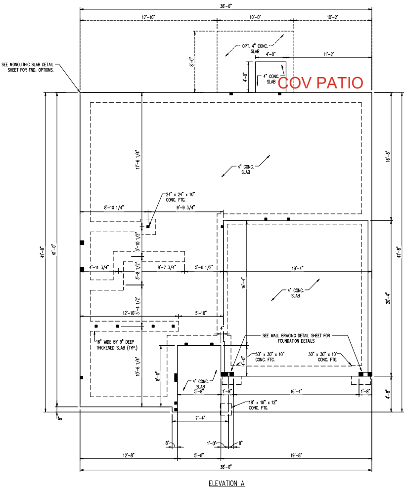
ELEVATION A
