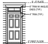
ENTRY DETAIL "B" SCALE: 1/8" = 1'-0"
