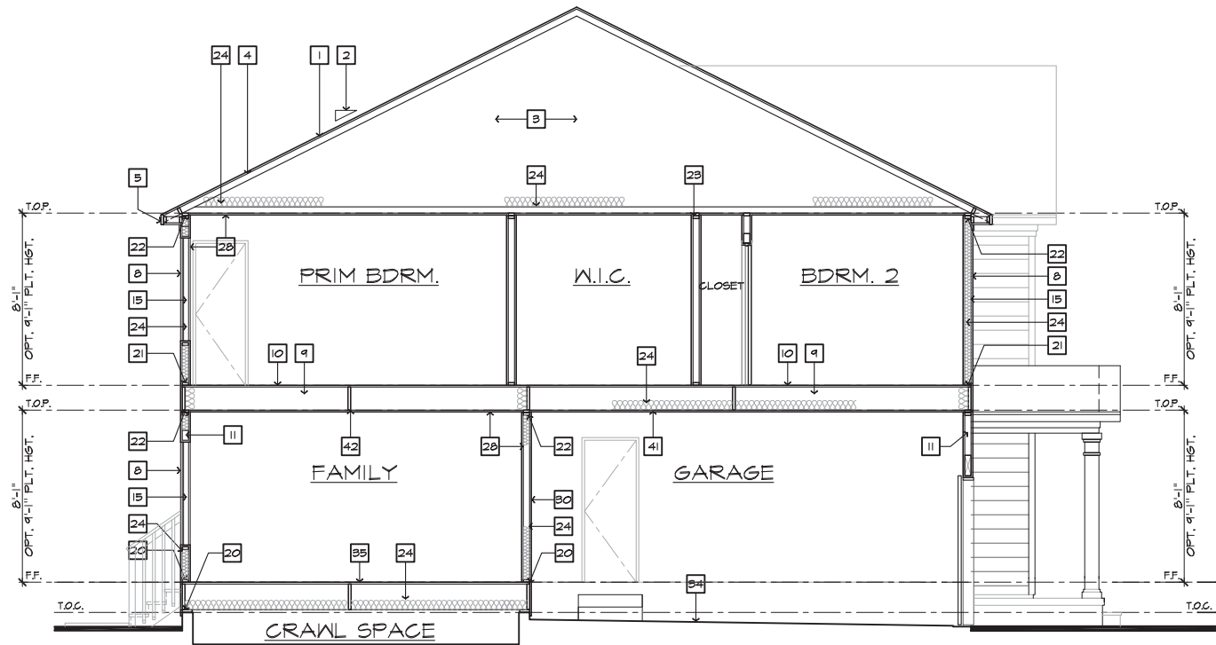
SECTION 'B'
