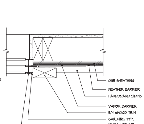
WINDOW JAMB
