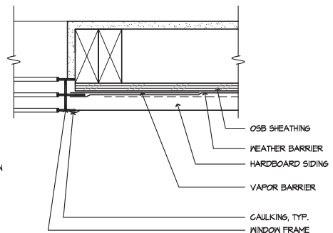
WINDOW JAMB
