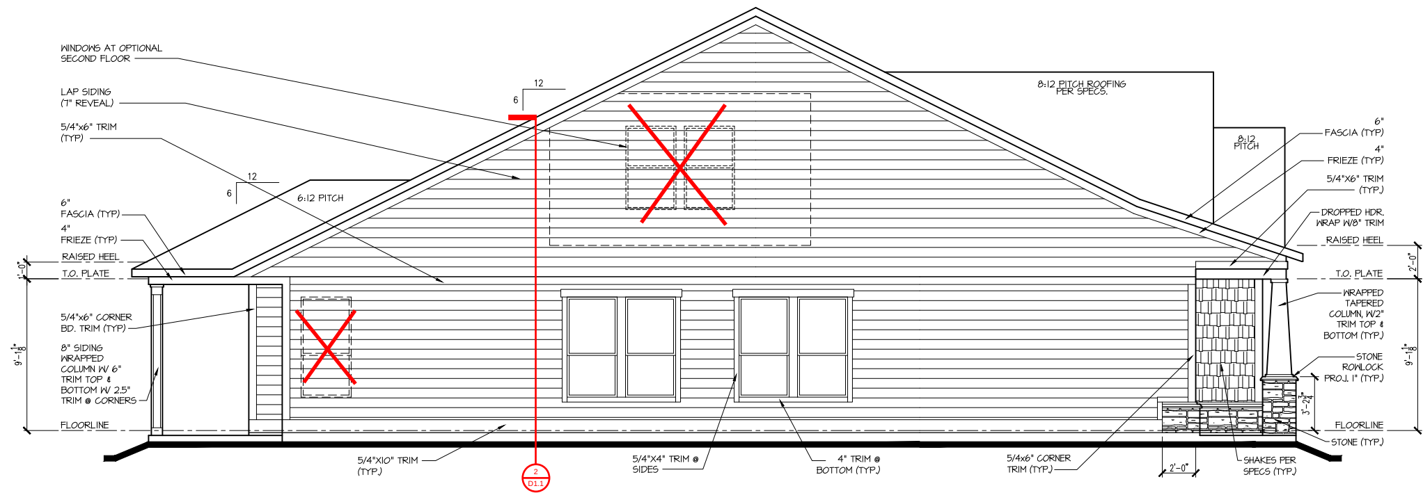
LEFT ELEV. "C" 1/8"=1'-0"
