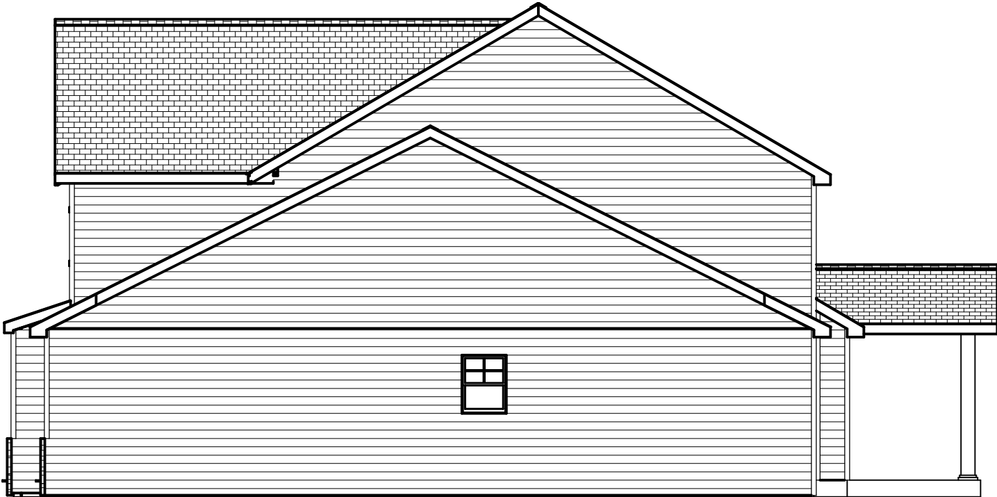
RIGHT ELEVATION
