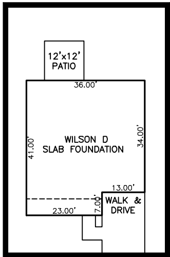
INSET SCALE: 1"=30"
