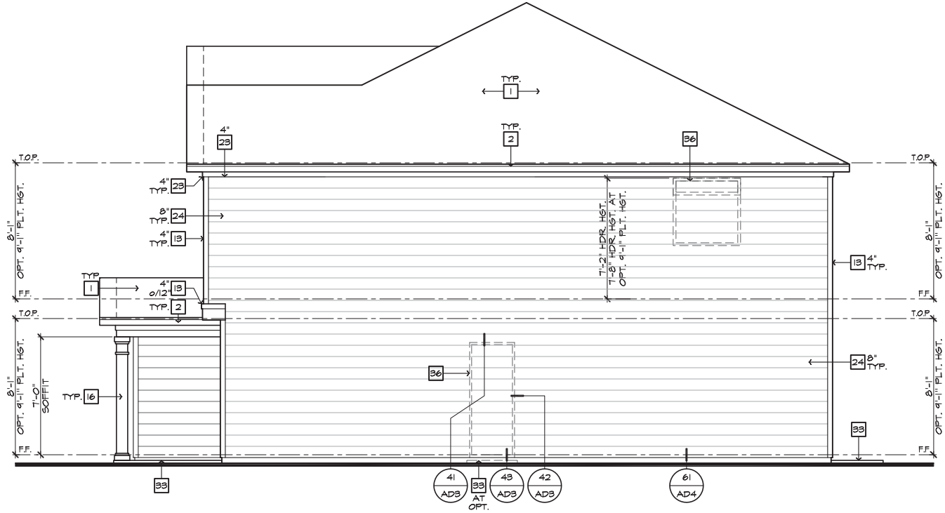
RIGHT ELEVATION 'L'
