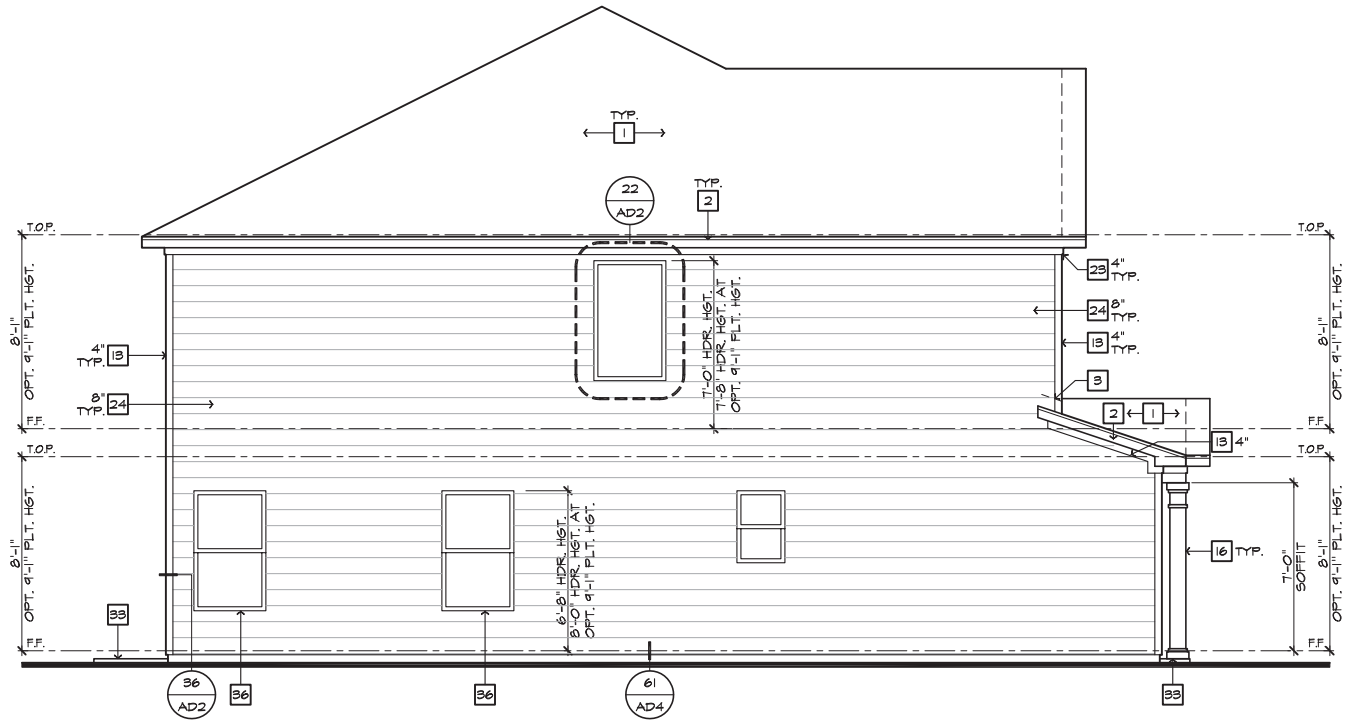
LEFT ELEVATION 'L'
