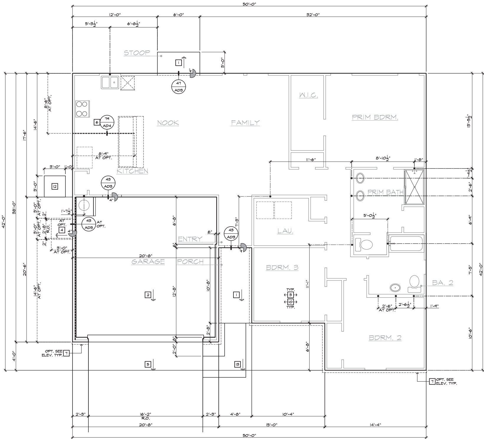
SLAB INTERFACE PLAN 'L'
