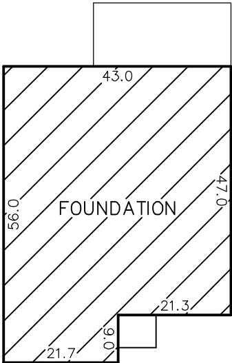
INSET N.T.S
