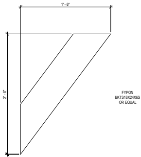
BRACKET DETAIL "B" SCALE: 1" = 1'-0"
