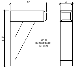
BRACKET DETAIL "A" SCALE: 1" = 1'-0"
