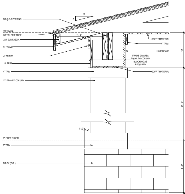
CORNICE DETAIL SCALE: 1" = 1'-0"
