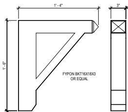
BRACKET DETAIL SCALE: 1" = 1'-0"
