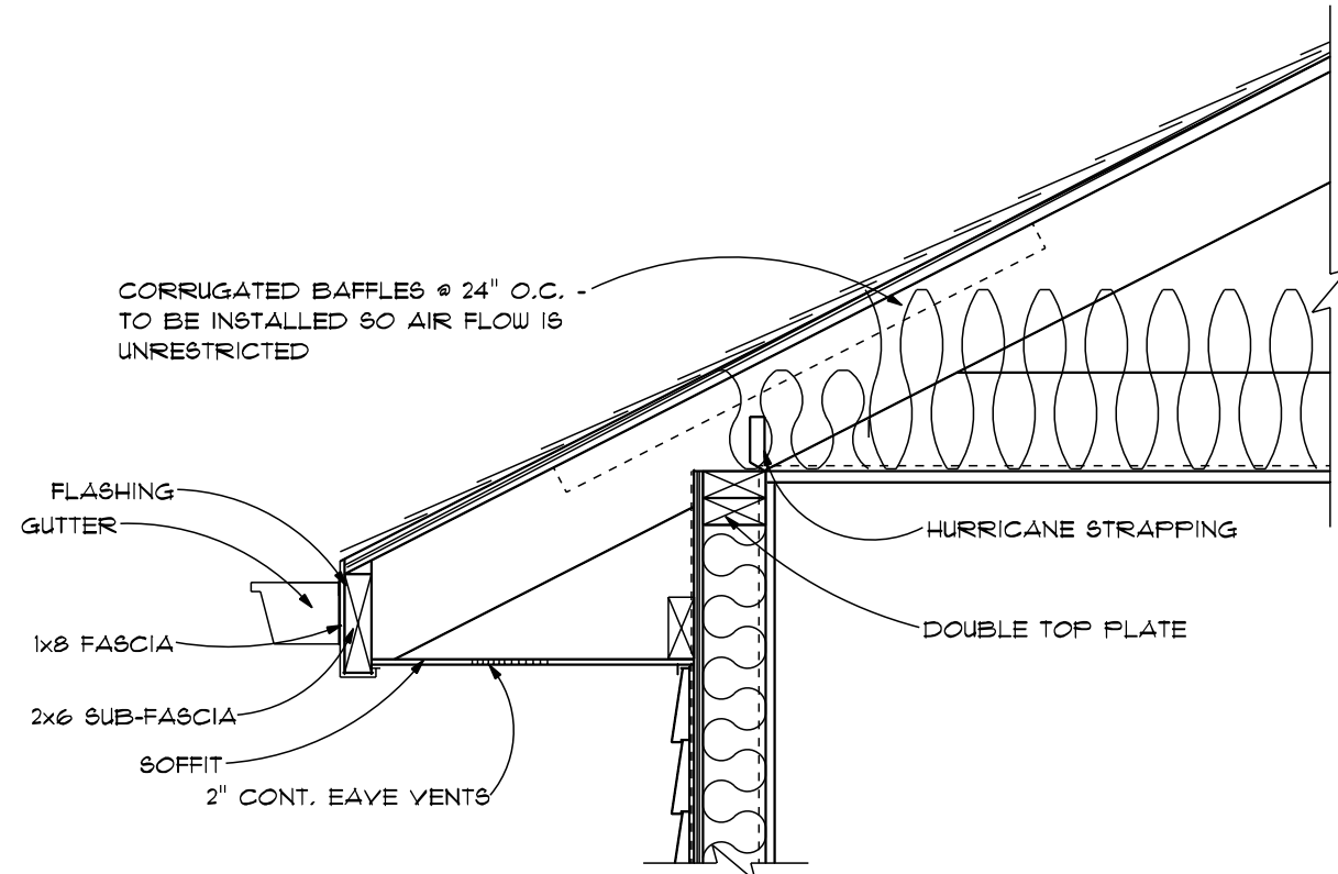
EAVE VENT
