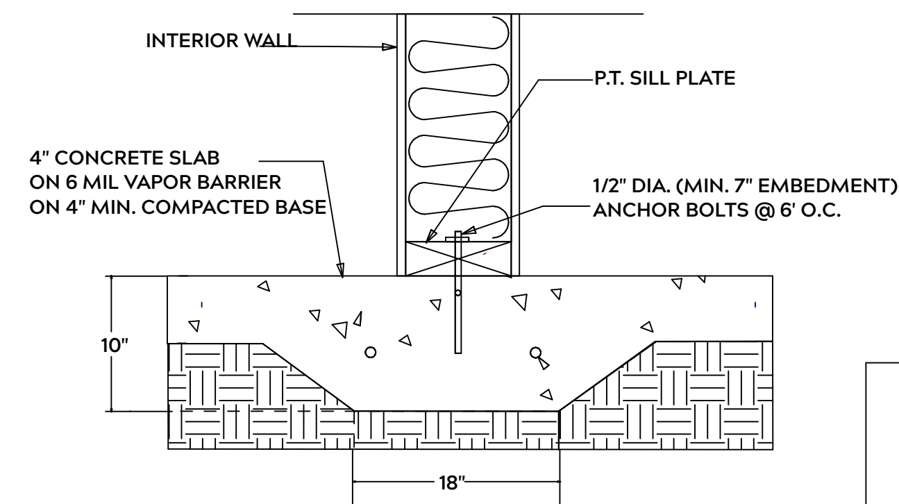
LUG FOOTING
