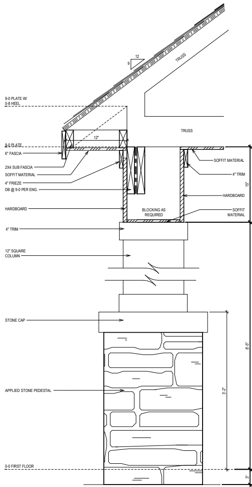
CORNICE DTL.
