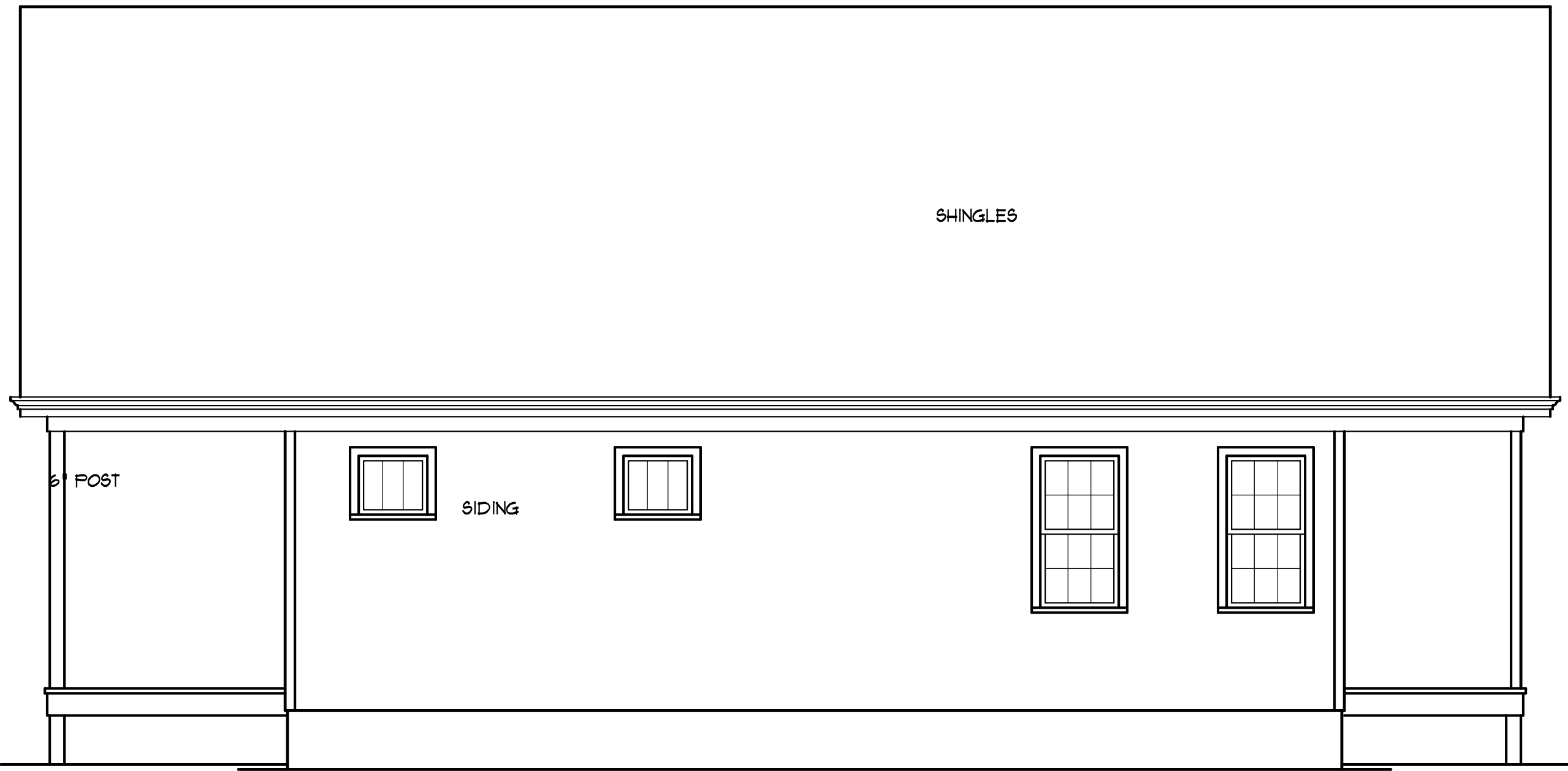
RIGHT SIDE ELEV SCALE: 1/4" = 1'-0"
