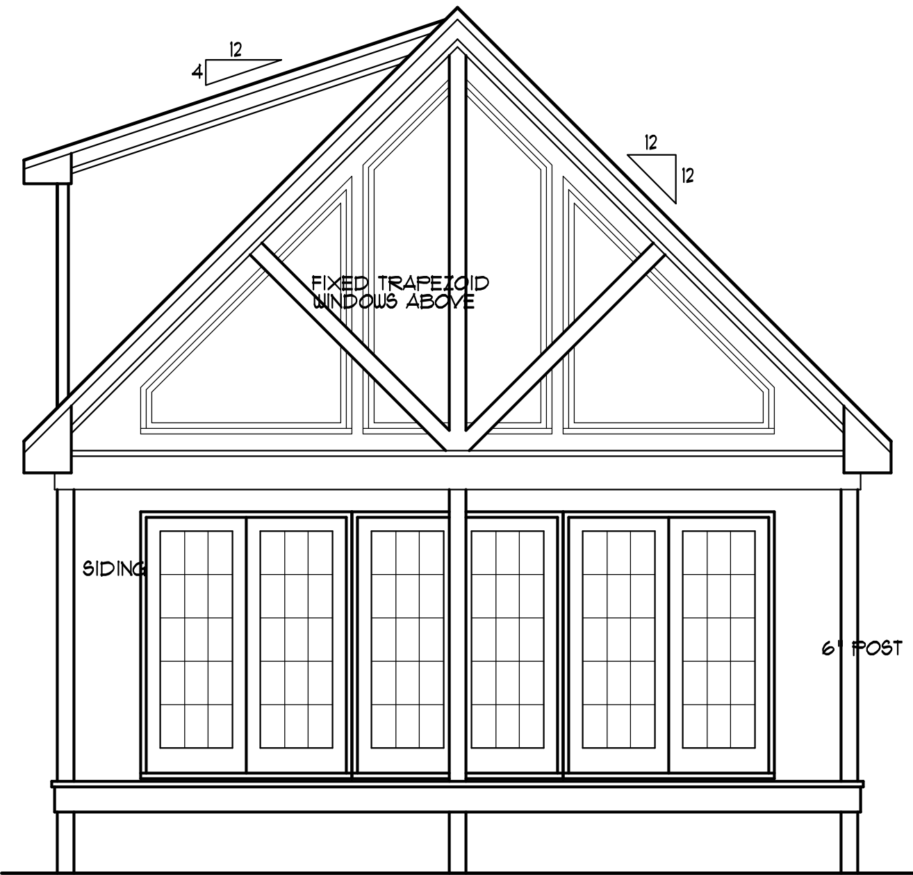
FRONT ELEV SCALE: 1/4" = 1'-0"
