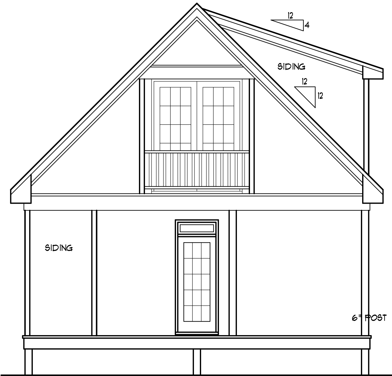
REAR ELEV SCALE: 1/4" = 1'-0"
