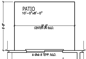
OPT PATIO SCALE: 1/4" = 1'-0"
