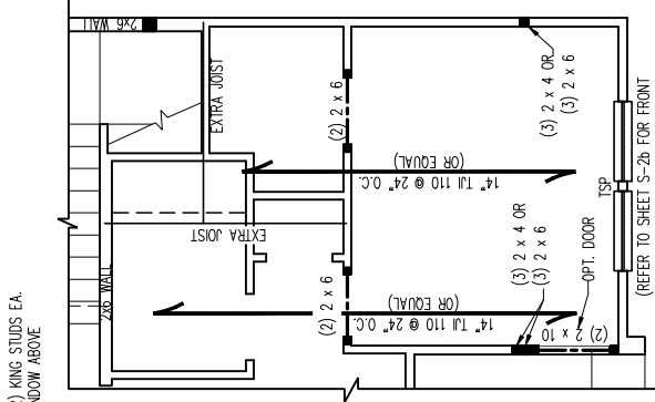
OPTIONAL BEDROOM 5 / BATH 3
