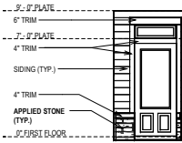
ENTRY DOOR SCALE: 1/8" = 1'-0"
