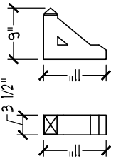
BRACKET DETAIL SCALE: 1/8" = 1'-0"
