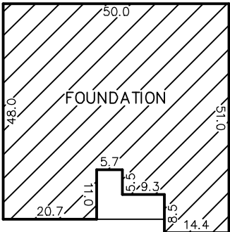
INSET N.T.S.
