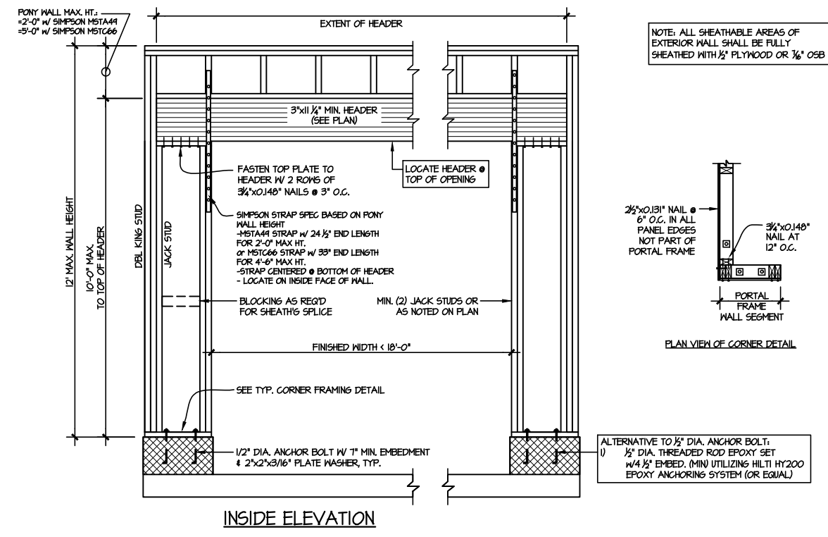
TWO SIDED GARAGE PORTAL FRAME BRACING ELEVATION ON CMU STEM 2 SCALE: N.T.S. SCALE: N.T.S.
