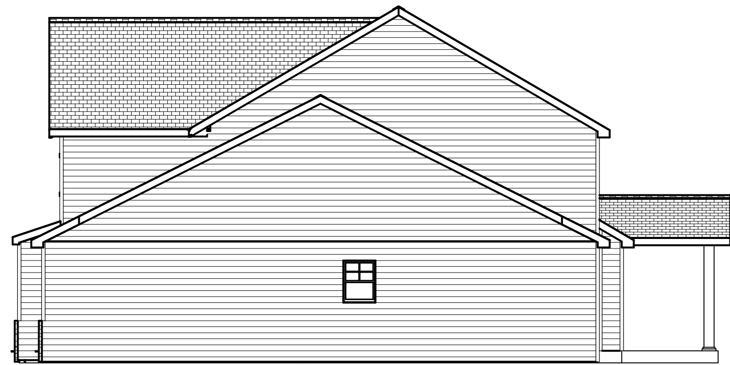
RIGHT ELEVATION
