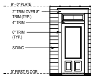
ENTRY DETAIL SCALE: 1/8" = 1'-0"
