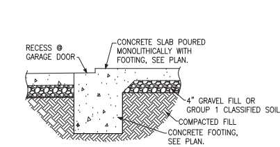
(G) GARAGE DOOR SECTION GARAGE DOOR
