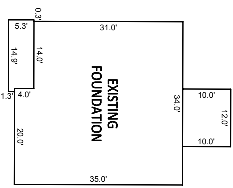
INSET SCALE: 1"=20'
