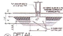
2 DETAIL SCALE: 3/4" = 1'-0"
