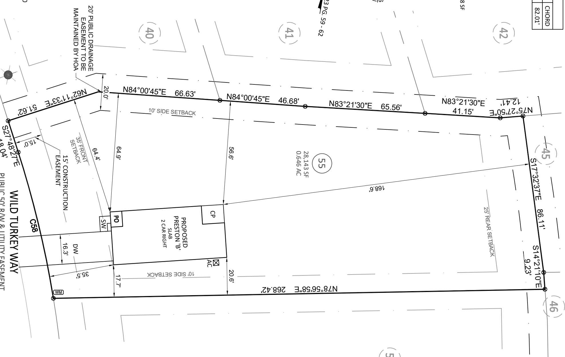
SCALE: 1" = 30 ft.
