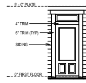
ENTRY DETAIL SCALE: 1/8" = 1'-0"
