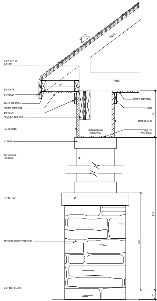
CORNICE DETL. SCALE: 1" = 1'-0"
