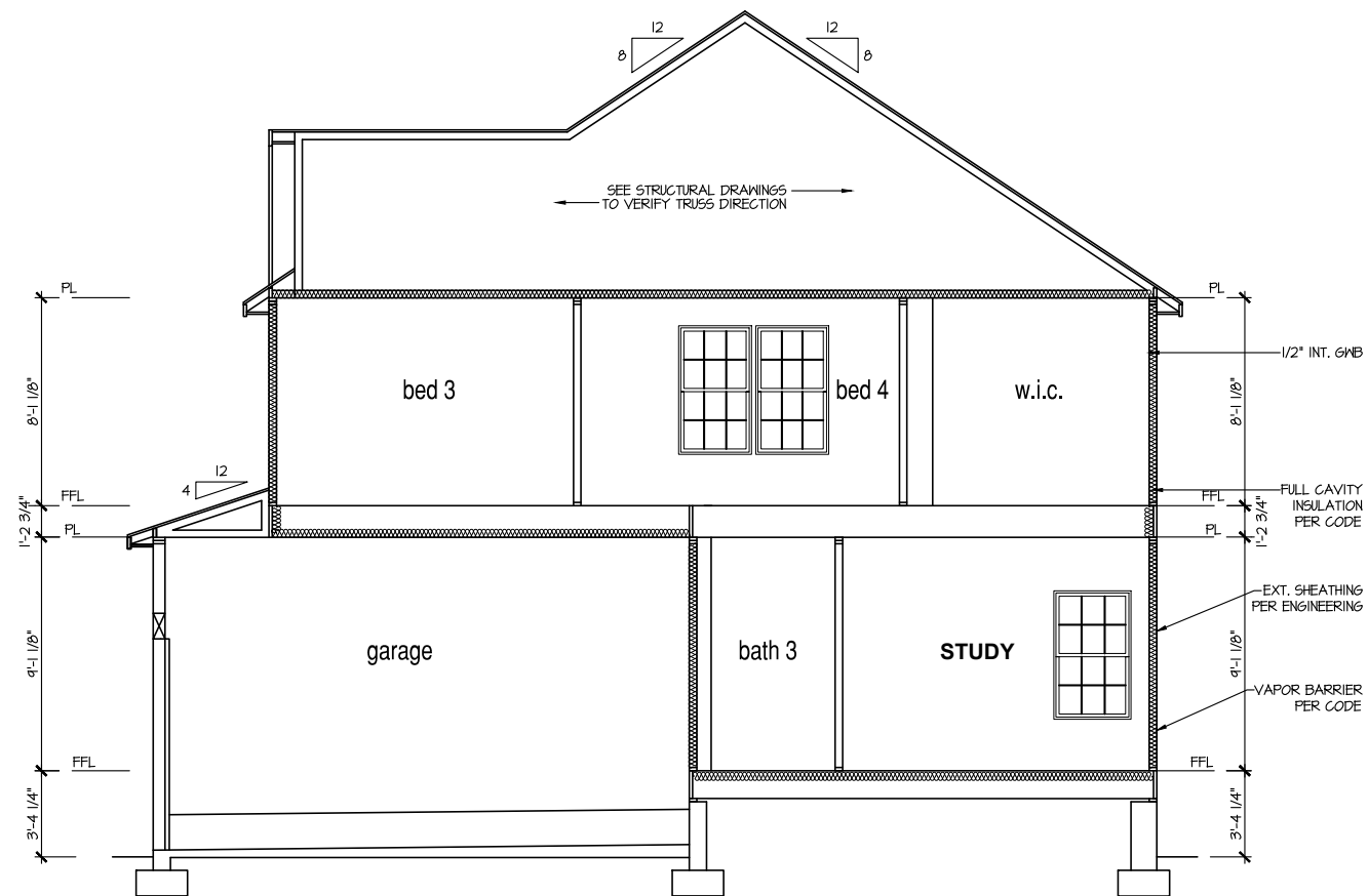
SECTION I SCALE: 1/8" = 1'-0"
