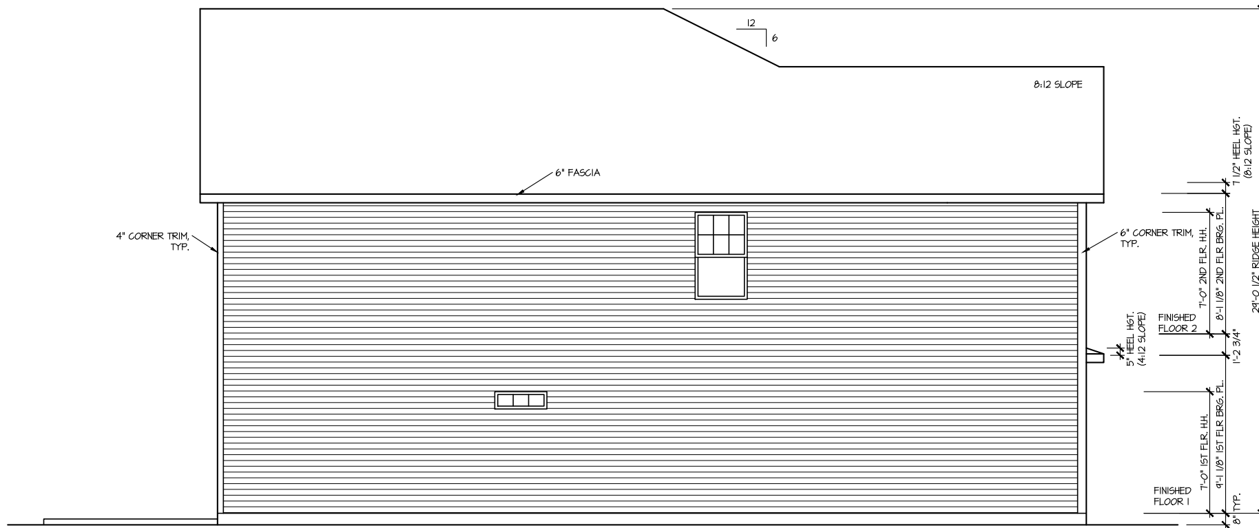
LEFT ELEVATION I
