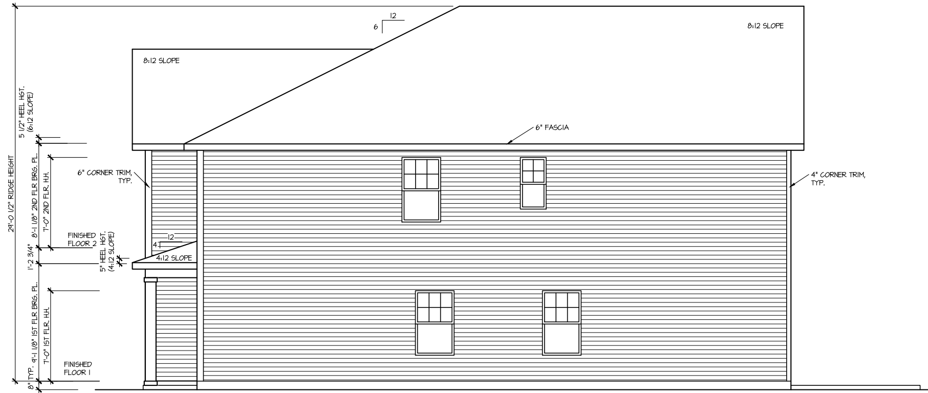
RIGHT ELEVATION I
