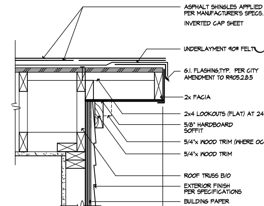
RAKE
