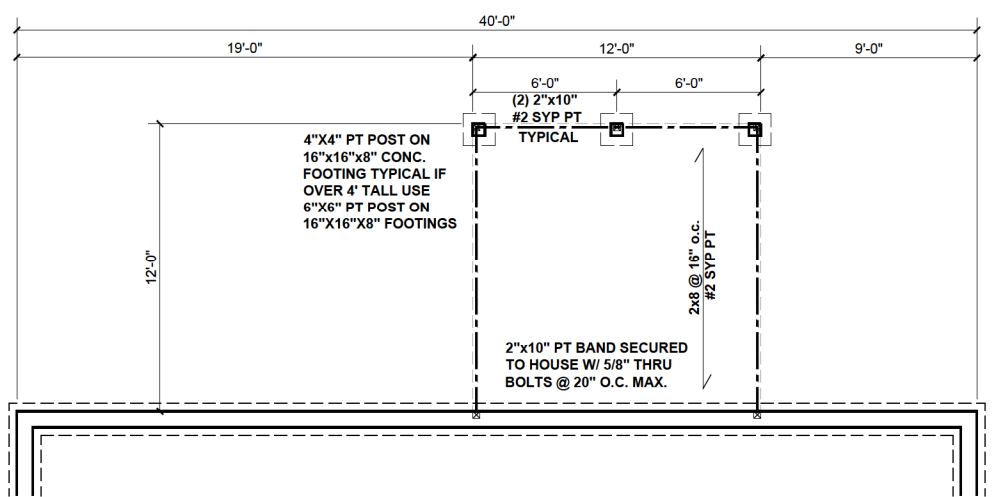
12' CRAWL FDN OPEN DECK SCALE: 1/8" = 1'-0"
