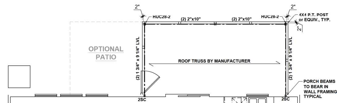
20'x10' SCREENED PATIO SCALE: 1/8" = 1'-0"
