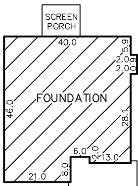
INSET N.T.S.
