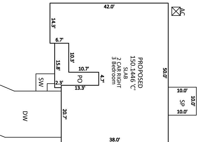
INSET SCALE: 1"=20'
