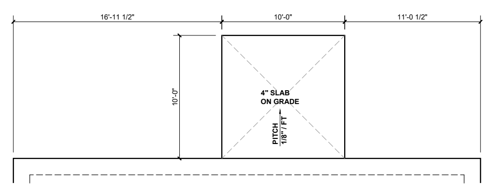
PATIO SLAB SCALE: 1/8" = 1'-0"
