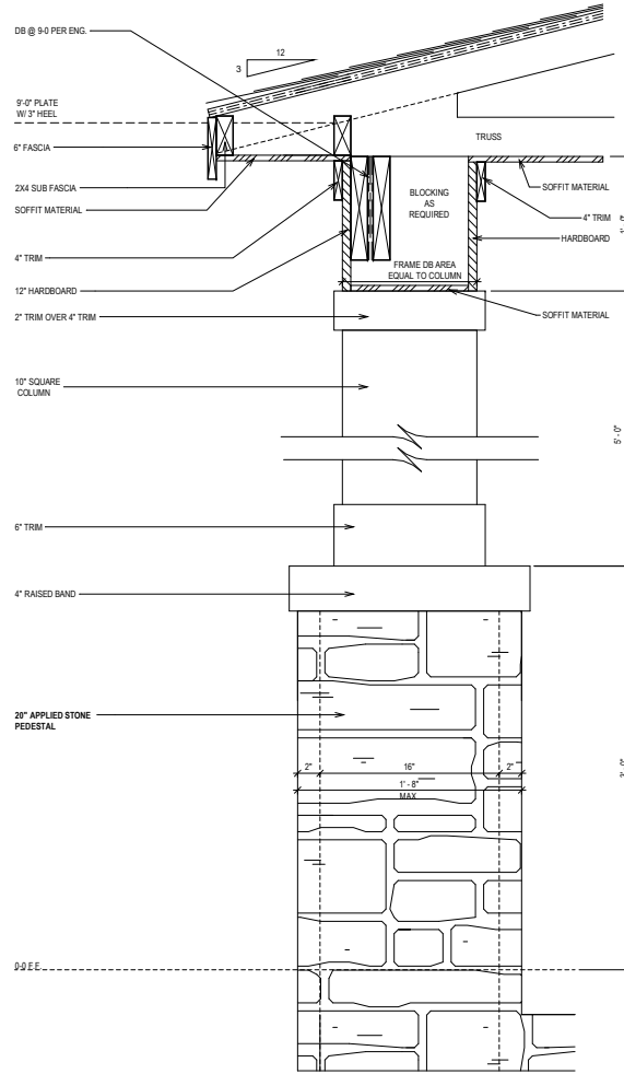
CORNICE A DETAIL SCALE: 1" = 1'-0"
