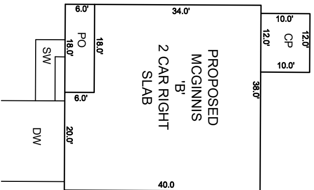
INSET SCALE: 1" = 20'
