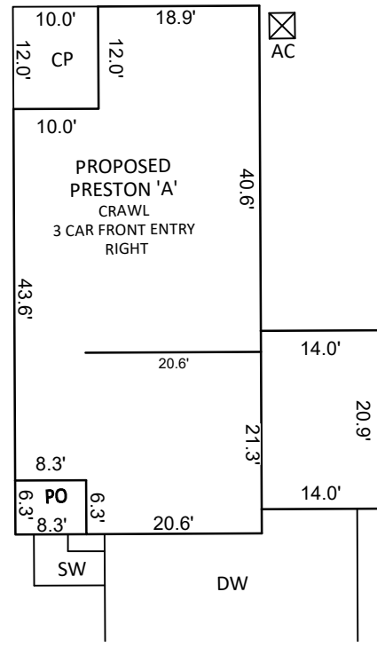
INSET SCALE: 1"=20'
