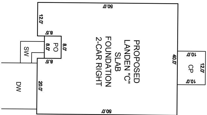
INSET SCALE: 1" = 20'
